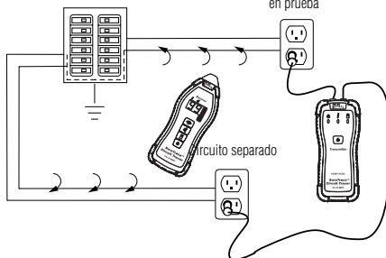
CONFIGURACIÓN DE SEÑAL INTENSA NO HAY CANCELACIÓN DE SEÑAL Circuito en prueba
